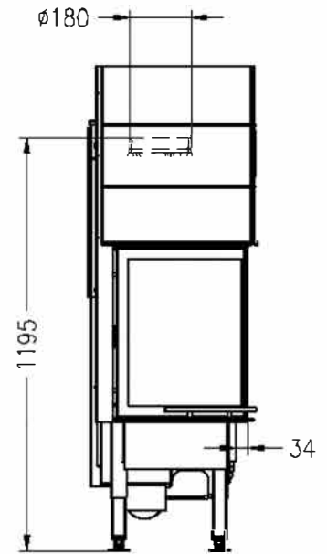
Seitenansicht M~1:20
